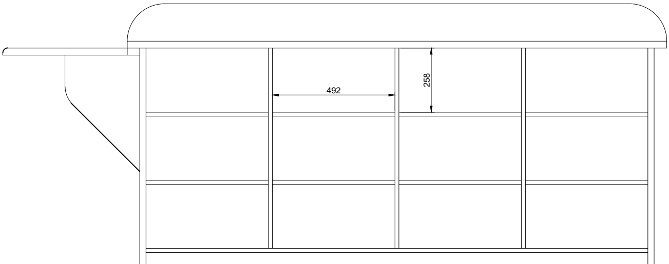
Skice Nr. 6 (skats no aizmugures)
