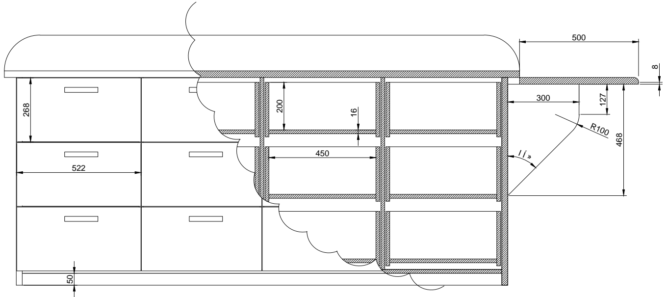
Skice Nr. 5 (skats no priekšpusēs ar griezumumu)
