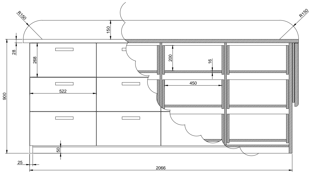
Skice Nr. 4 (skats no priekspuses ar griezumu)
